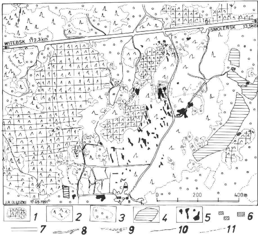
Ryc. 1. Las Katyński - 2.09.1942, (szkic fotointerpretacyjny). Objaśnienia: 1 — zwarte kompleksy leśne, 2 — kompleksy leśne o niewielkim zwarcu, 3 — obszary z pojedynczymi drzewami lub grupami drzew i krzaków, 4 — grunty orne, 5 — ślady potencjalnych wykopów, 6 — zabudowania, 7 — szosa, 8 — droga gruntowa, 9 — droga gruntowa o niewyraźnym przebiegu, 10 — ścieżka, 11 — ślad ścieżki. A — tzw. willa NKWD, spalona we wrześniu 1943; B — Budynek mieszkalny, zniszczony we wrześniu 1943; C — garaż, obiekt zachowany do końca roku 1990. Barwą czerwoną oznaczono naruszenia gruntu według stanu z dnia 14 października 1943 i z dnia 28 kwietnia 1944
